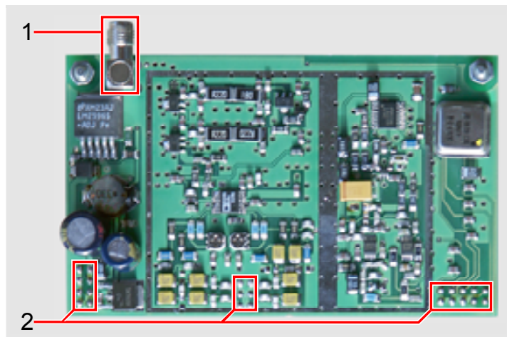
Abb. 2.1.a: Der IQ-Modulator
