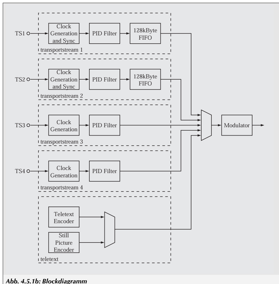
Abb. 4.5.1b: Blockdiagramm
